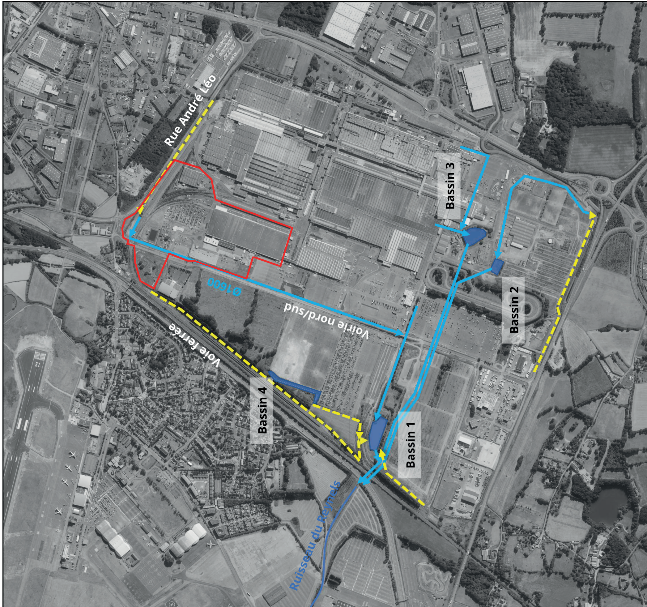
Schéma de principe du fonctionnement hydraulique à l'échelle du site industriel de La Janais
