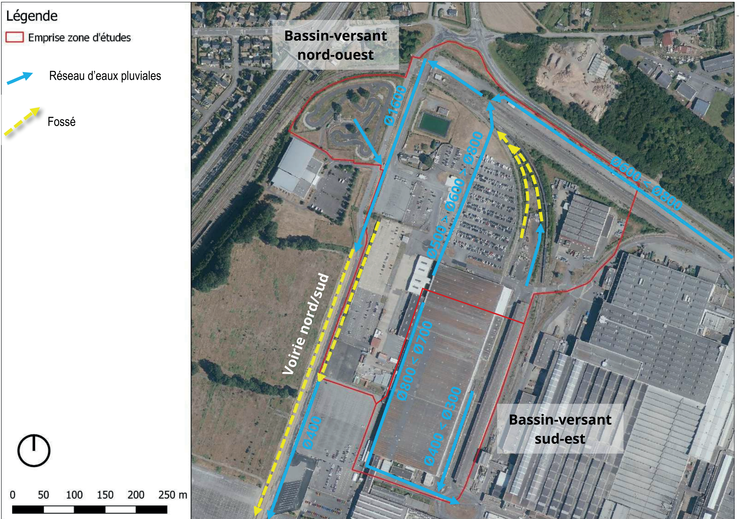
Figure 97 : Fonctionnement hydraulique au niveau du site d'études – IAO SENN, 2022
